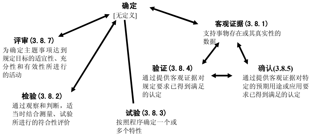
图 A11 有关检查的概念 (3.8)
