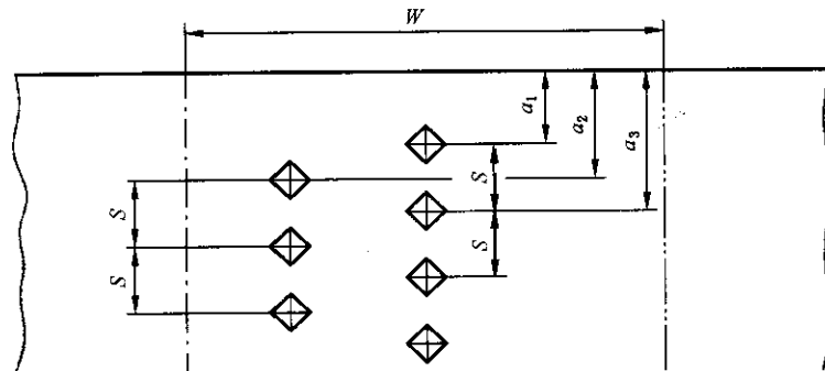
图 1 硬度压痕的位置
