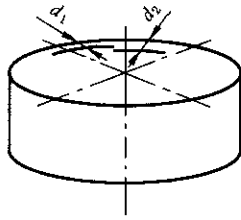
图2 硬度测量点的位置
