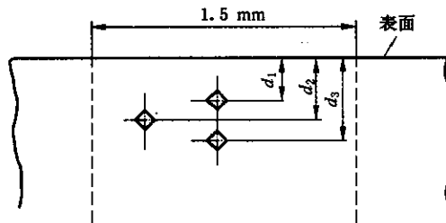
图 1 硬度压痕的位置
