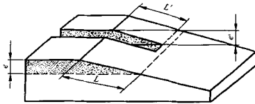
图 3 有槽的斜截面试样
