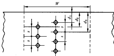
图5 显微硬度压痕的定位
