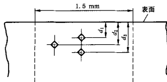
图 1 硬度压痕的位置
