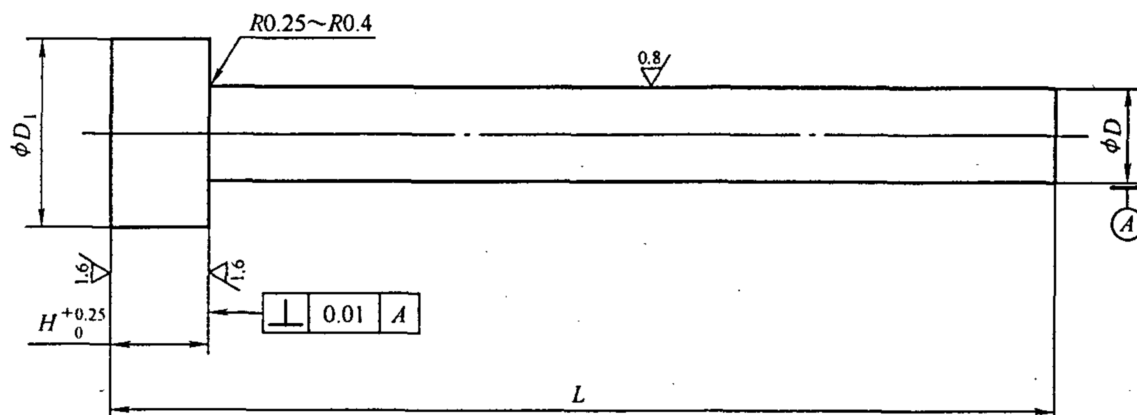
图 1 圆柱头直杆圆凸模
