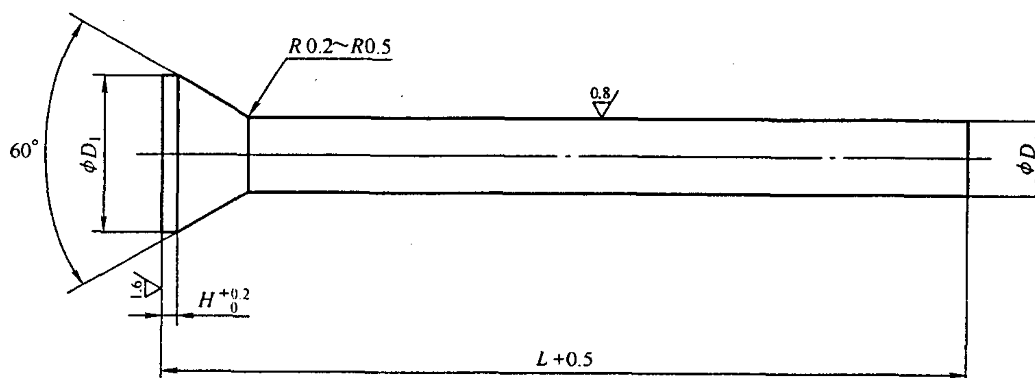
图 1 60° 锥头直杆圆凸模
