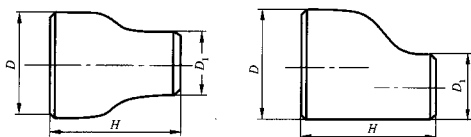
图 10 异径接头
