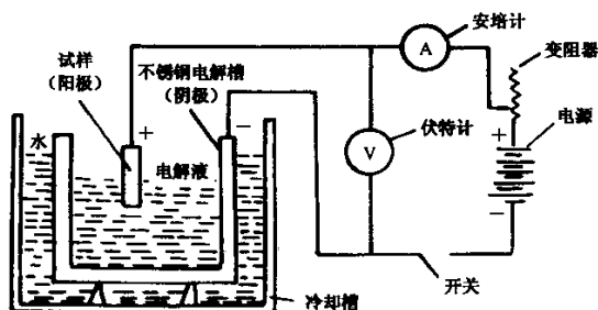
图1 电解抛光装置示意图
