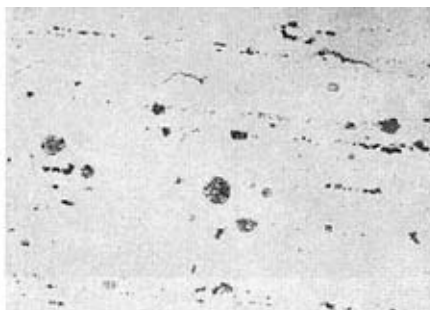
图 16 2A12(LY12)合金棒材淬火过烧组织 3号浸蚀剂浸蚀 ×200
