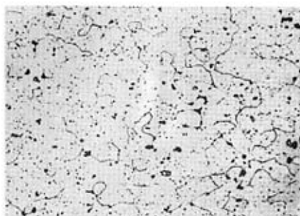
图 18 7A04(LC4)合金型材淬火过烧 3号浸蚀剂浸蚀 ×200
