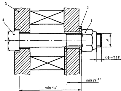
1—螺母试件;2—试验垫圈 2) ;3—试验装置;4—试验螺栓
