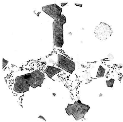
图5 严重过烧组织
