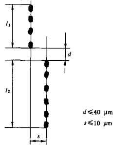
图9 B类夹杂物
