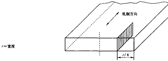
图4 厚度 \leq 25 mm钢板的取样
