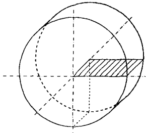
图 2 直径或边长 > 25 mm ~ 40 mm 钢棒或钢坯的取样
