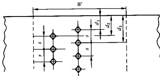
图 5 显微硬度压痕的定位
