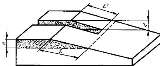
图 3 有槽的斜截面试样
