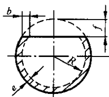
图 1 机械加工平面得到的纵截面试样
